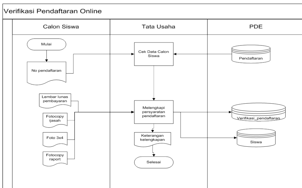
Gambar 4.2 Sistem Flow Pendaftaran Siswa Via Online
