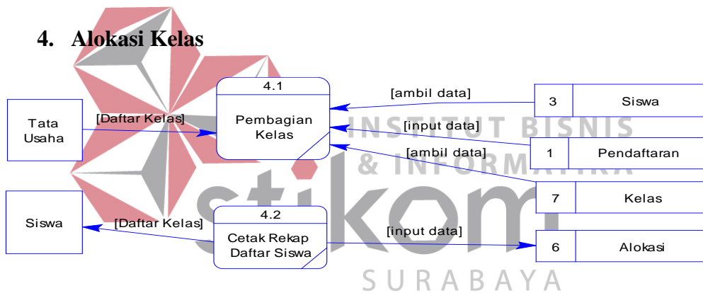
Gambar 4.12 Level 1 Alokasi Kelas
