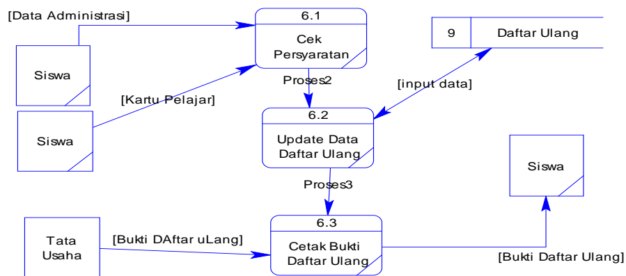
Gambar 4.13 Level 1 Daftar Ulang
