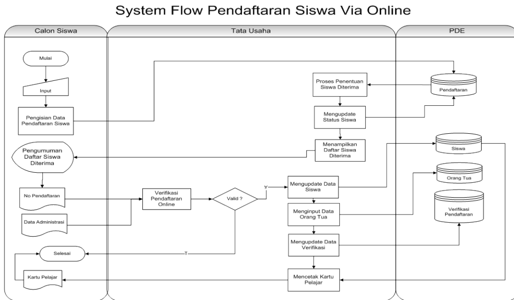
Gambar 4.1 Sistem Flow Pendaftaran Siswa Mutasi
