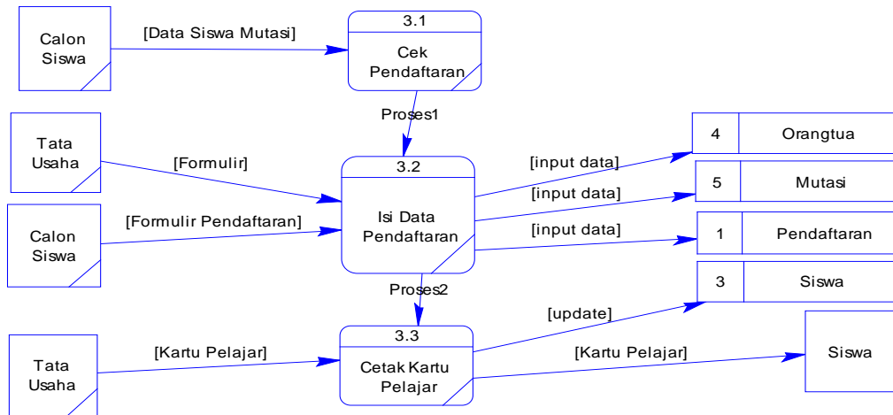
Gambar 4.11 Level 1 Pendaftaran Siswa Mutasi
