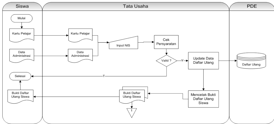
Gambar 4.4 Sistem Flow Pendaftaran Siswa Mutasi
