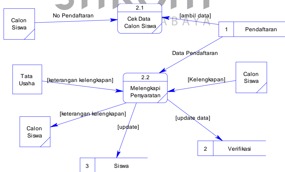
Gambar 4.10 Level 1 Verifikasi Pendaftaran
