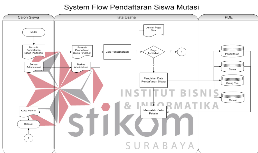
Gambar 4.3 Sistem Flow Pendaftaran Siswa Mutasi
