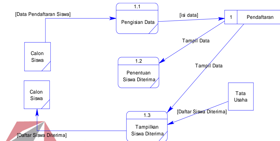
Gambar 4.9 Level 1 Pendaftaran Siswa Baru Online
