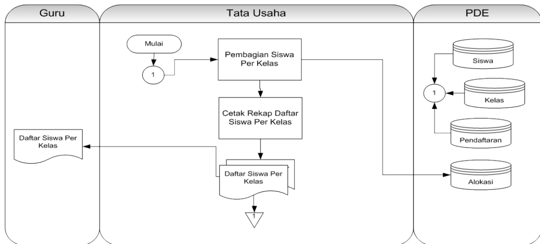
Gambar 4.5 Sistem Flow Alokasi Kelas
