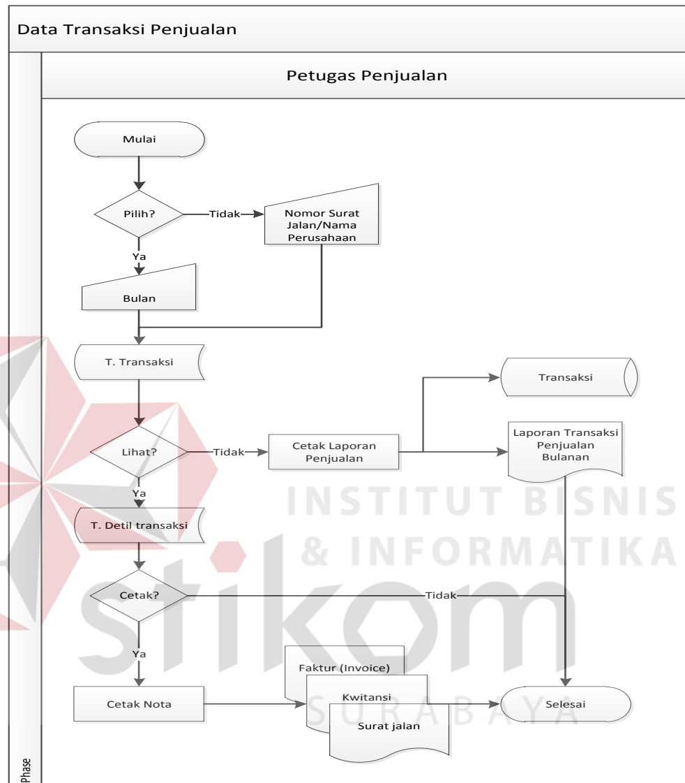
Gambar 4.3 Data Transaksi Penjualan
