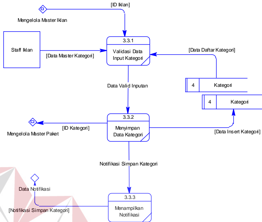
Gambar 4.15 DFD Level 2 Mengelola Master Kategori
