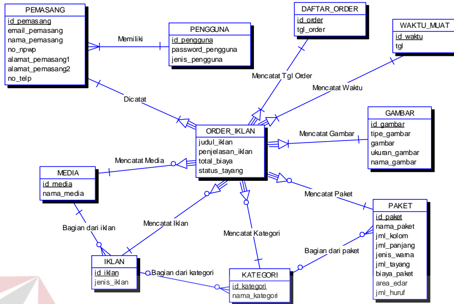
Gambar 4.22 ERD CDM Aplikasi Order Iklan
