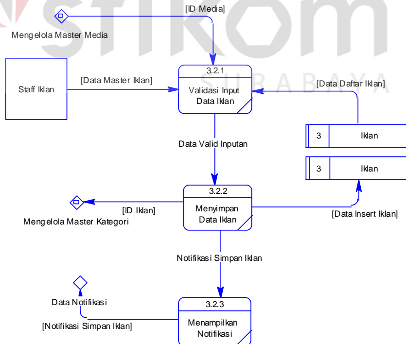
Gambar 4.14 DFD Level 2 Mengelola Master Iklan
