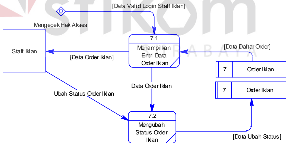
Gambar 4.20 DFD Level 1 Mengelola Order Iklan
