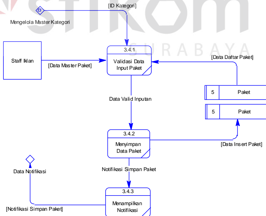
Gambar 4.16 DFD Level 2 Mengelola Master Paket
