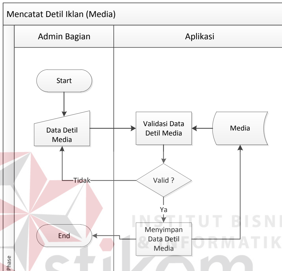
Gambar 4.2 System Flow Detil Iklan (Media)
