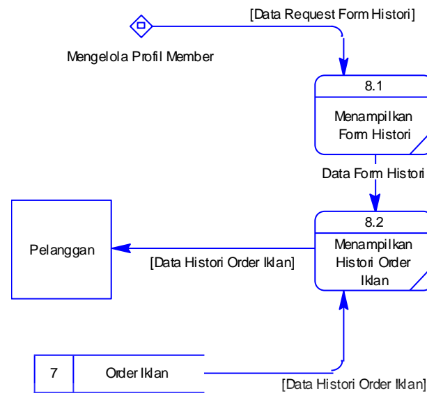
Gambar 4.21 DFD Level 1 Melihat Histori Order Iklan
