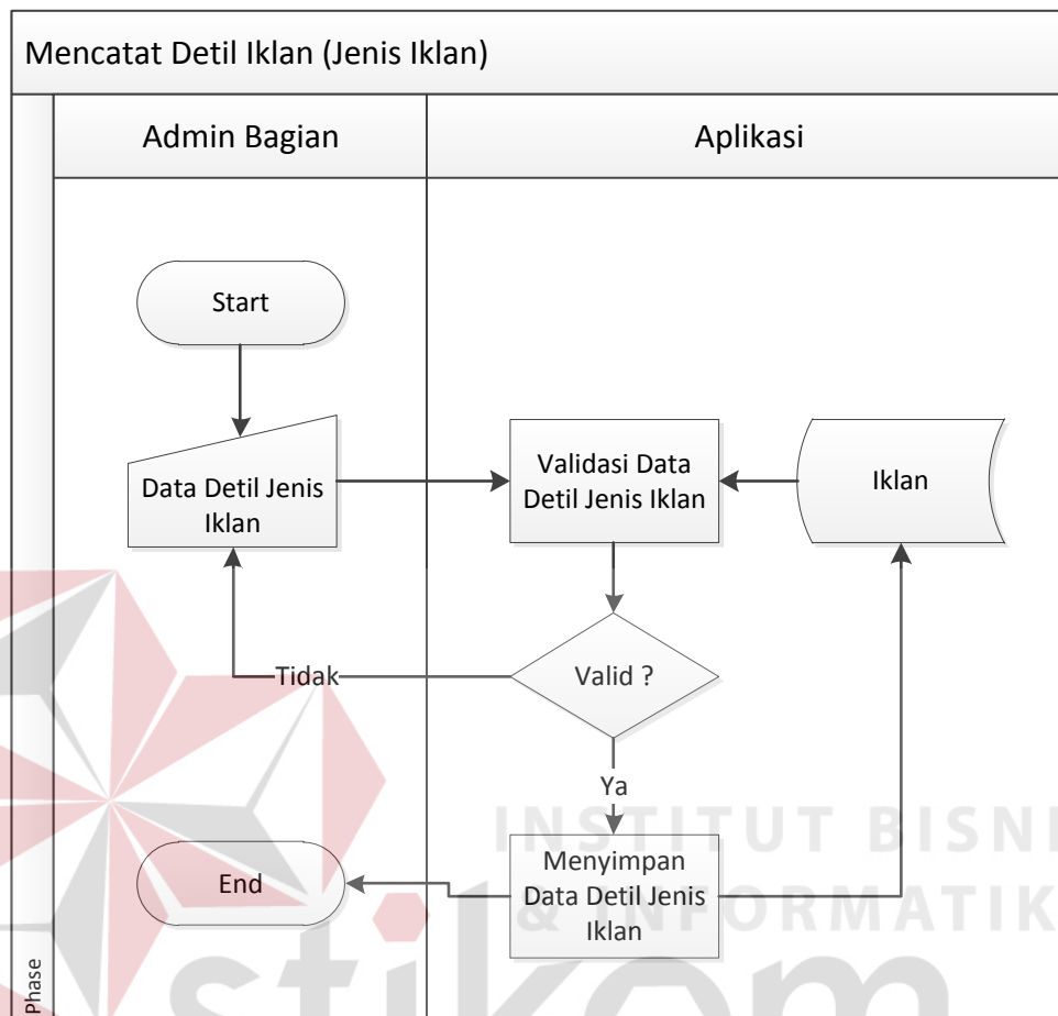
Gambar 4.3 System Flow Detil iklan (Jenis iklan)
