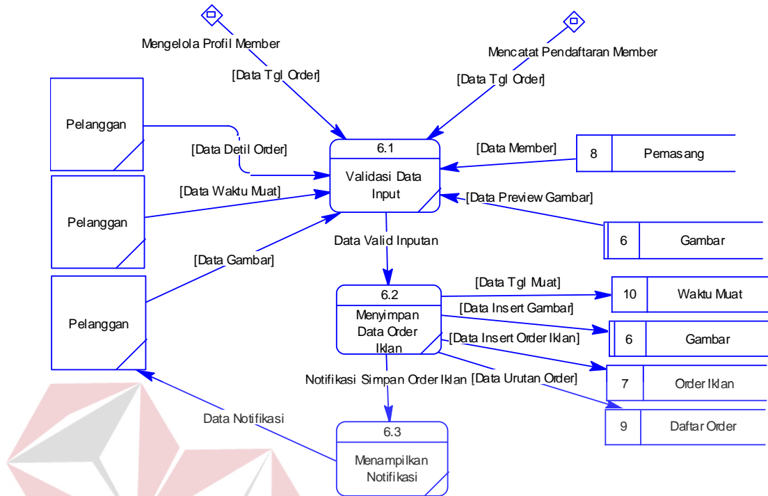
Gambar 4.19 DFD Level 1 Mencatat Order Iklan
