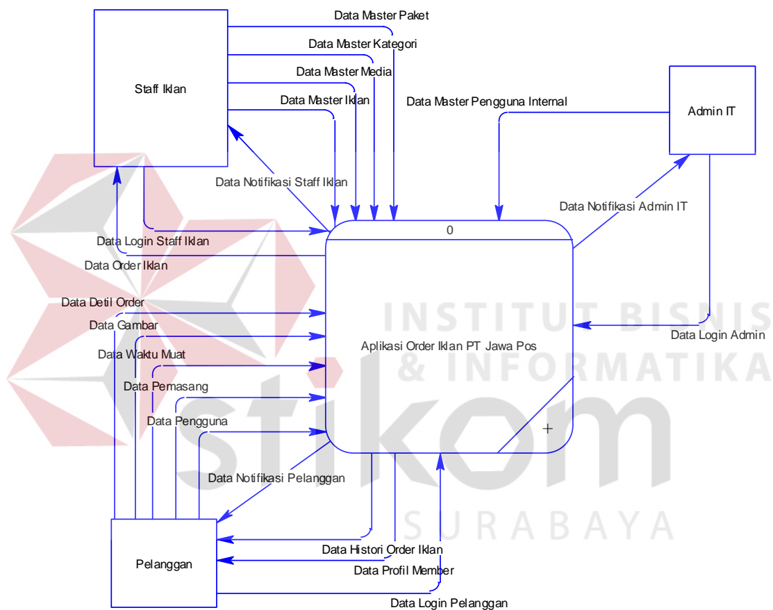
Gambar 4.8 Context Diagram Aplikasi Order Iklan
