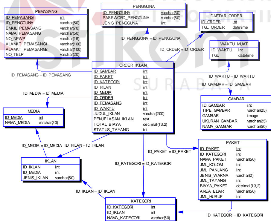
Gambar 4.23 ERD PDM Aplikasi Order Iklan
