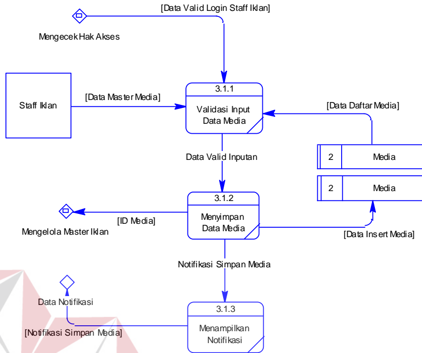
Gambar 4.13 DFD Level 2 Mengelola Master Media
