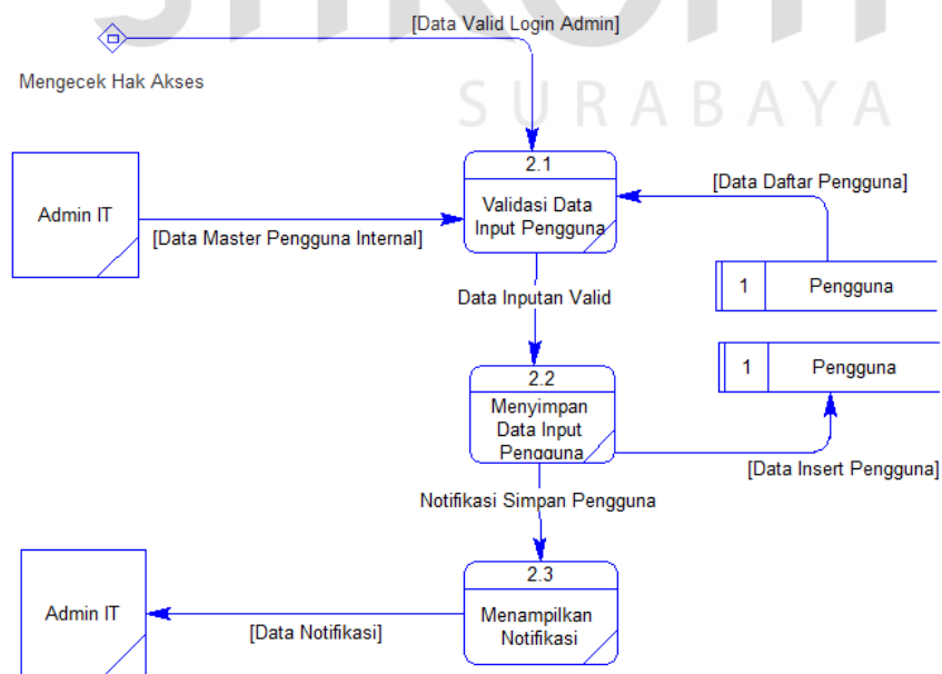
Gambar 4.11 DFD Level 1 Mengelola Master Pengguna
