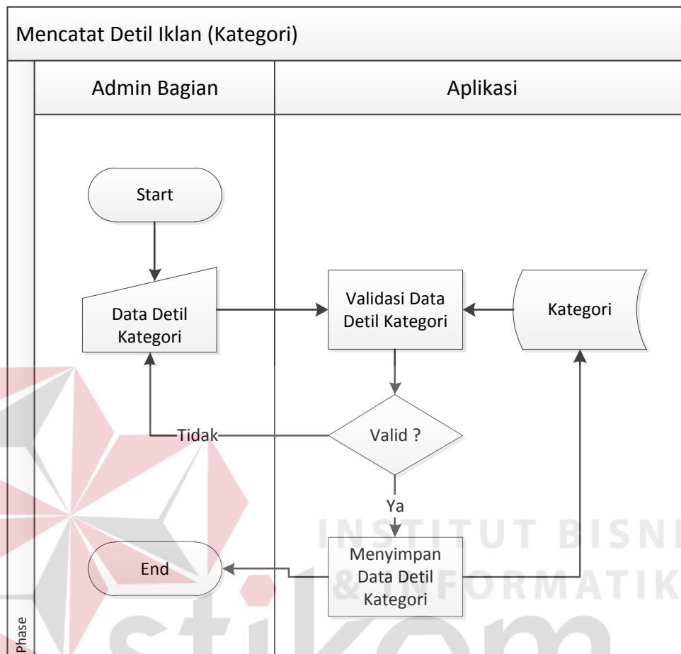
Gambar 4.4 System Flow Detil Iklan (Kategori)
