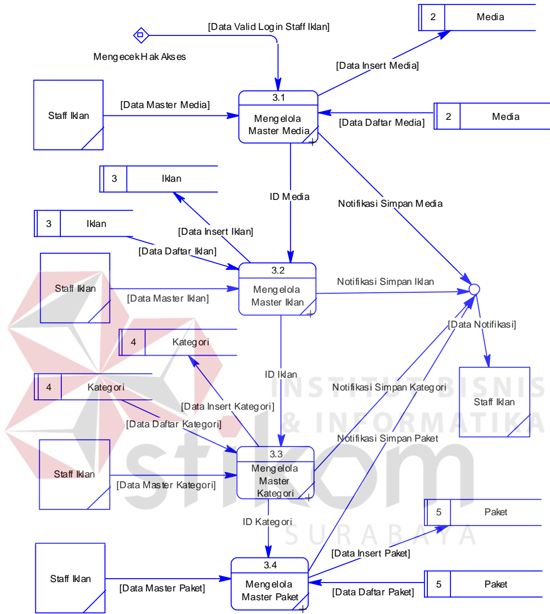
Gambar 4.12 DFD Level 1 Mengelola Master Detil Iklan
