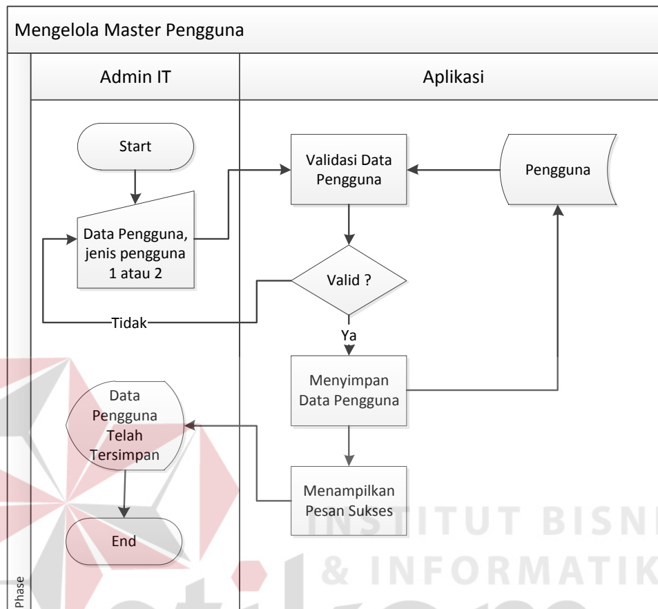
Gambar 4.1 System Flow Master Pengguna
