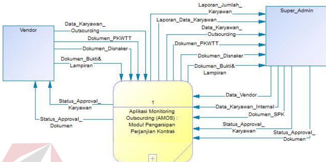
Gambar 4.11 Context Diagram Pengarsipan Perjanjian Kontrak
