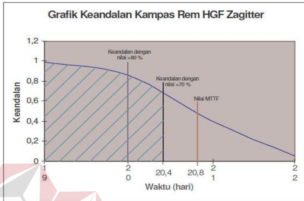
Gambar 4.4. Grafik Keandalan Kampas Rem HGF Zagitter
