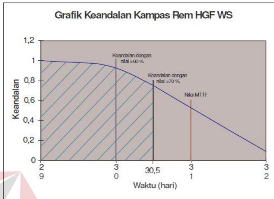
Gambar 4.2. Grafik Keandalan Kampas Rem HGF WS
