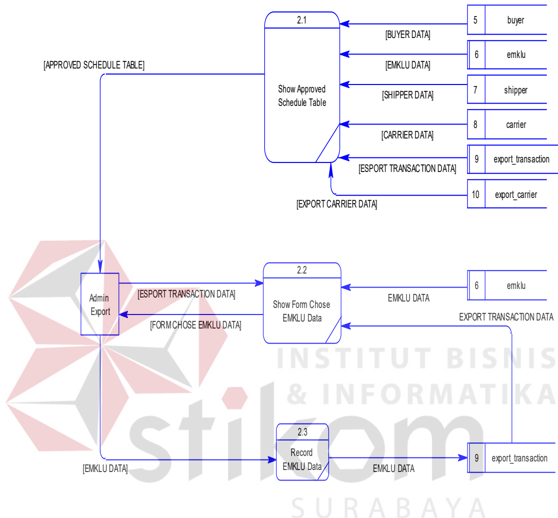
Gambar 4.21 Data flow diagram level 1 set EMKL atau EMKU
