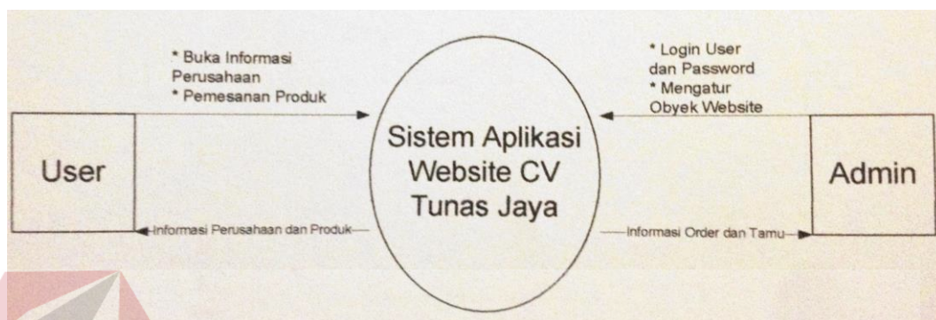
Gambar 4.13 : Diagram Konteks
