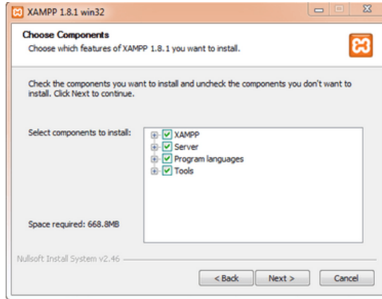
Gambar 4.3. Fitur Xampp
