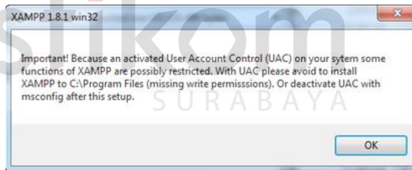
Gambar 4.2. UAC windows
