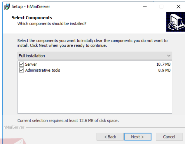
Gambar 4.8. Komponen hmailserver
