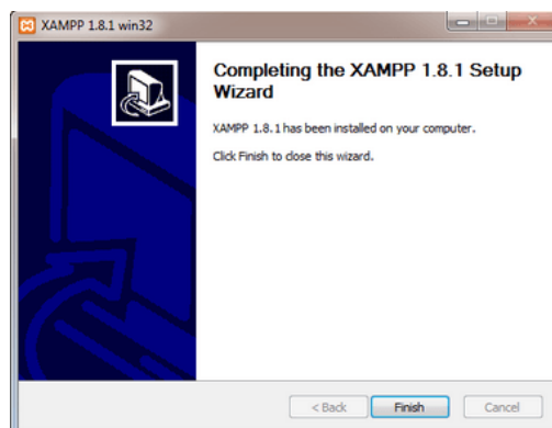
Gambar 4.5. Instalasi Selesai
