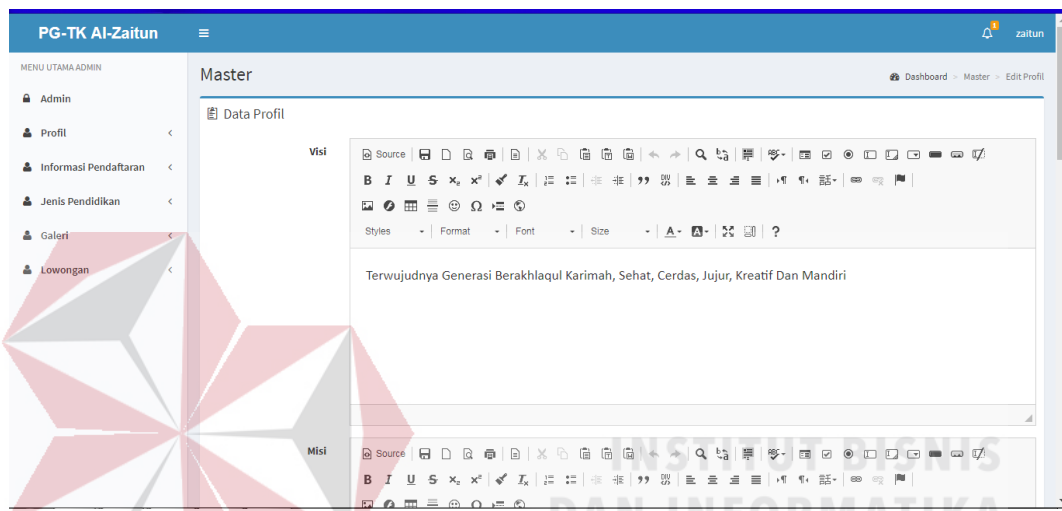
Gambar 1. 14 Admin Profil
