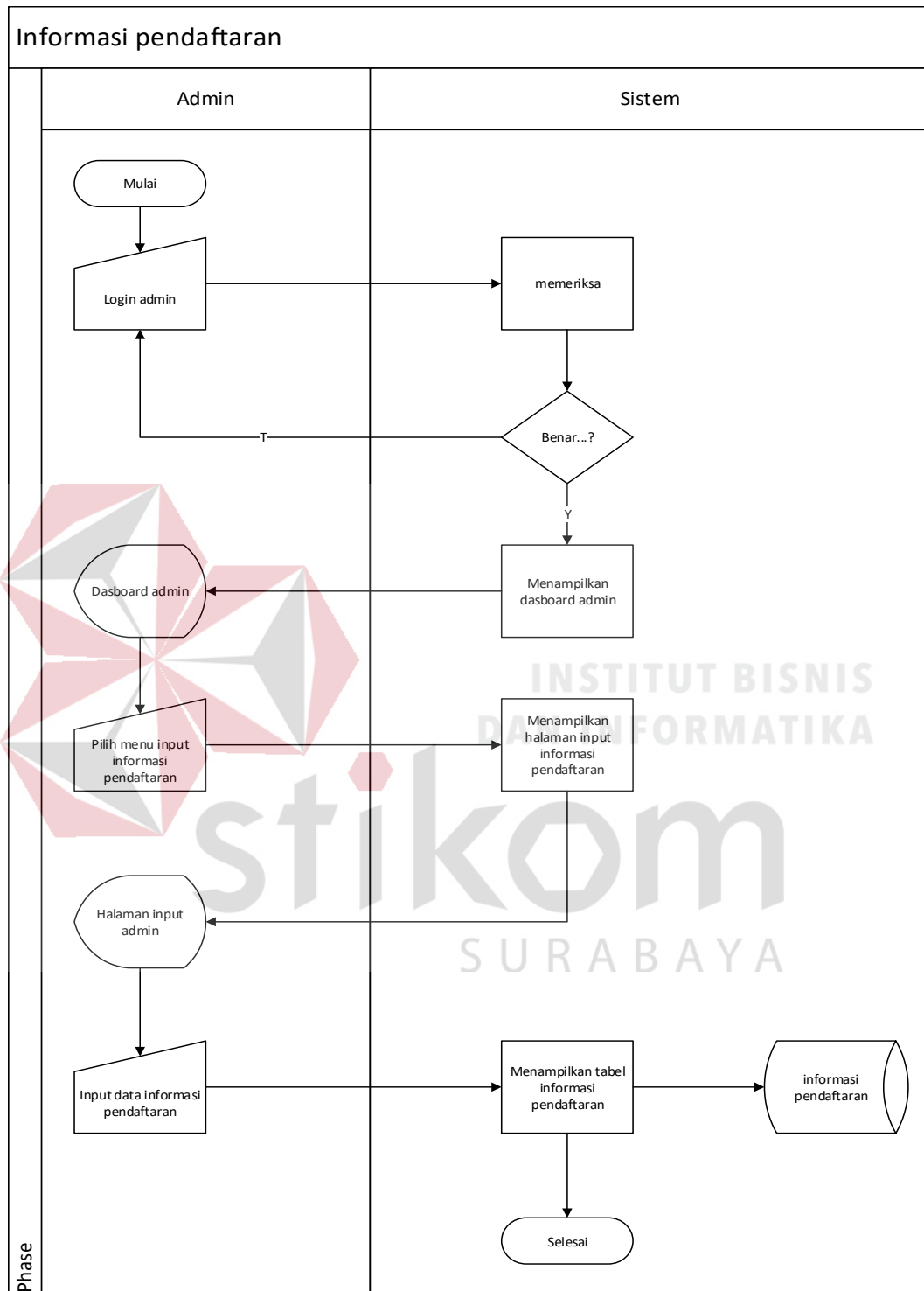
Gambar 1.3 Sistem Flow Maintenance Data Informasi Pendaftaran
