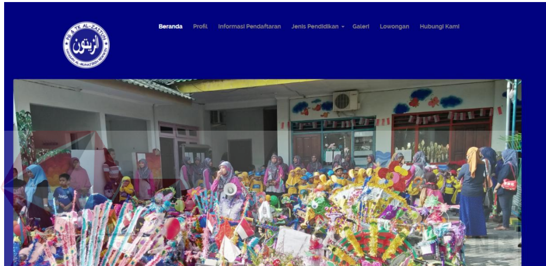
Gambar 1. 1 Tampilan Beranda
