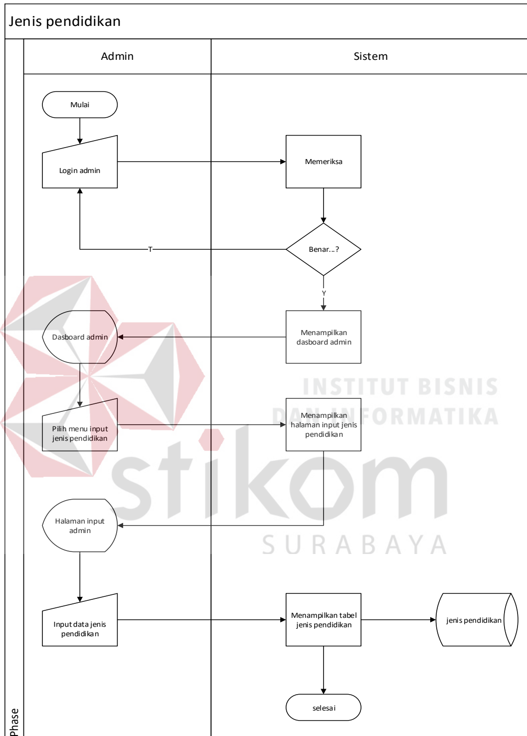
Gambar 1. 4 Sistem Flow Maintenance Jenis Pendidikan
