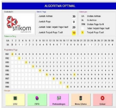
Gambar 6. Hasil Pengujian Algoritma Optimal
