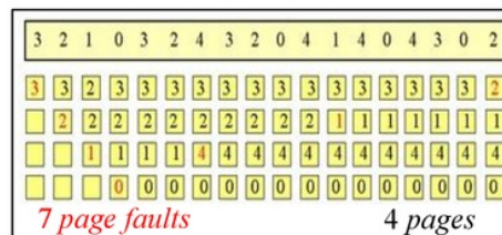
Gambar 2. Page Replacement Algoritma Optimal dengan 4 Page .
