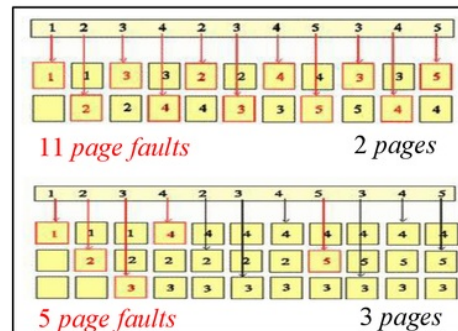
Gambar 1. Page Replacement Algoritma FIFO dengan 2 Page dan 3 Page .
