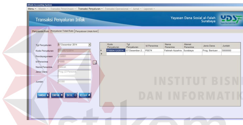
Gambar 4.66 Hasil Uji Tampilan Datagridview Penyaluran Infak/Sedekah
