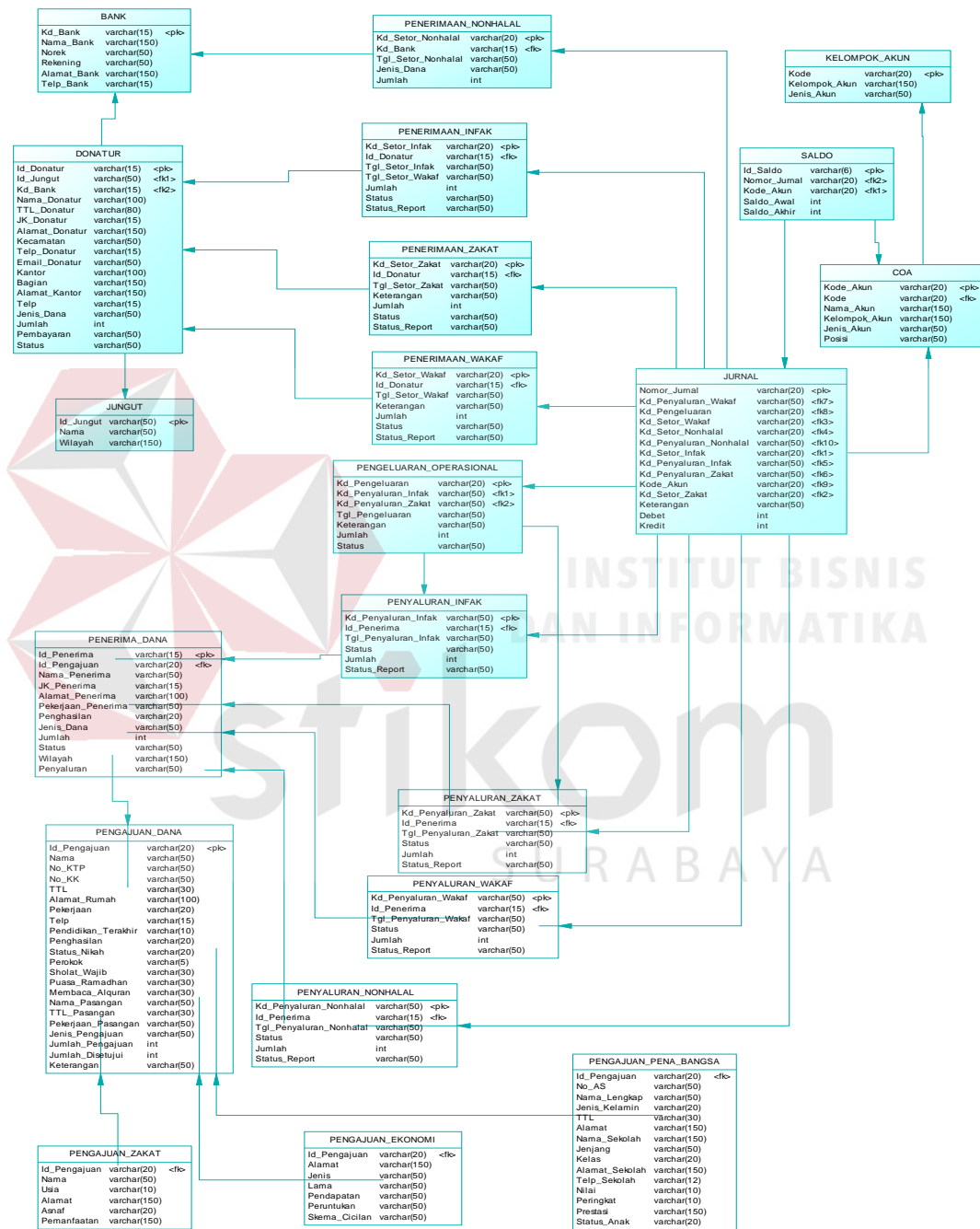
Gambar 3.25 PDM Rancang Bangun Aplikasi Pembuatan Laporan Keuangan Berdasarkan PSAK 109 Pada YDSF
