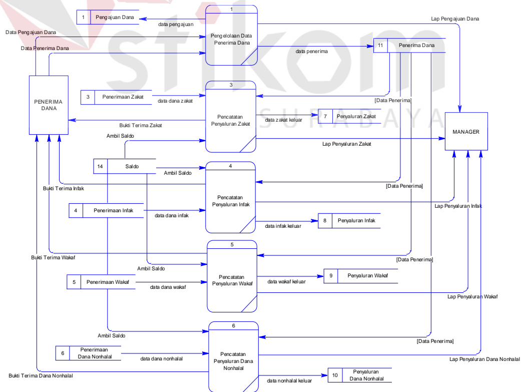
Gambar 3.21 DFD Level 1 Penyaluran Dana
