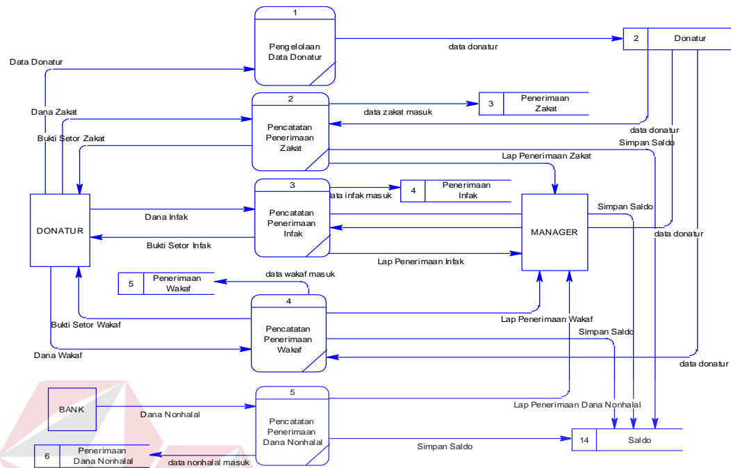
Gambar 3.20 DFD Level 1 Penerimaan Dana
