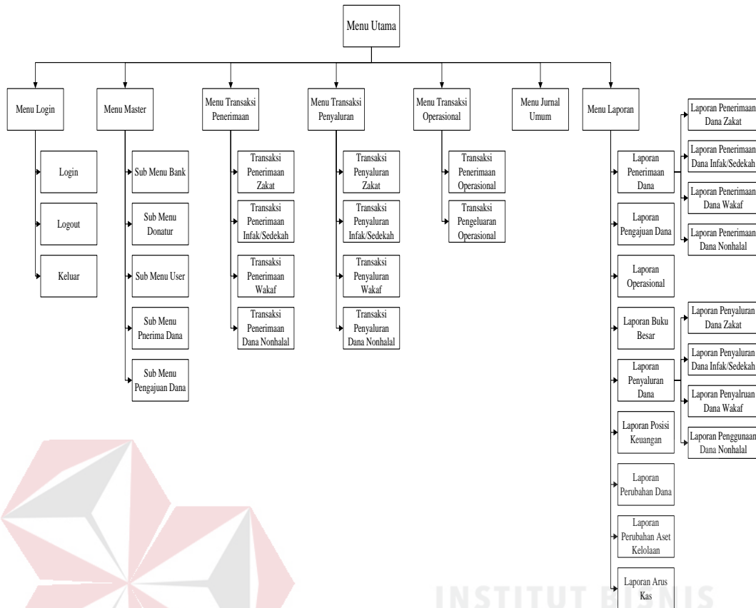
Gambar 3.47 Diagram Menu Utama dan Sub Menu
