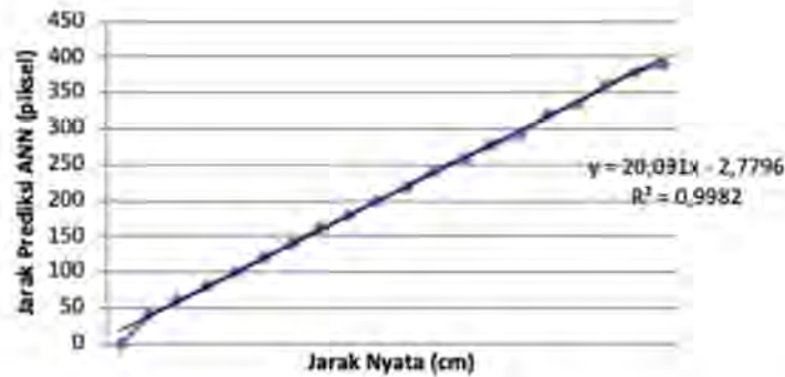
Gambar 12. Hubungan Antara Nilai Jarak Prediksi ANN Terhadap Jarak Nyata
