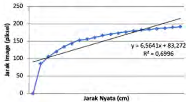
Gambar 10. Grafik Nilai Jarak Terhadap Jarak Nyata
