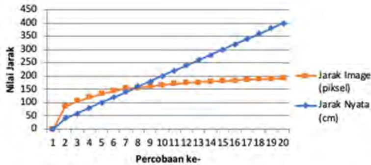
Gambar 9. Grafik Nilai Jarak Terhadap Data Percobaan
