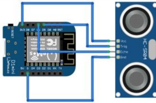
2 Gambar 5. Rangkaian Sensor Ultrasonik HC-SR04
