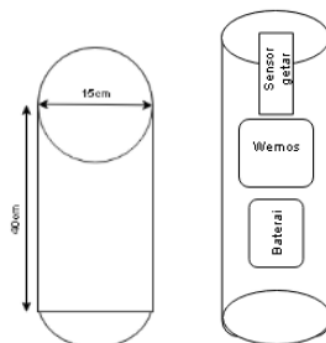
Gambar 9. Perancangan Patok Tiang Pembatas Sensor Getar
