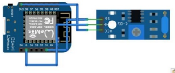
Gambar 3. Rangkaian Sensor Getar SW-420
