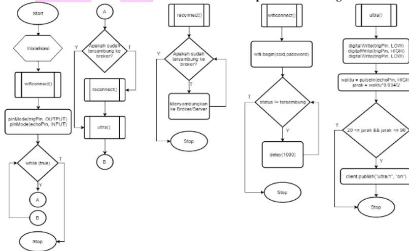
Gambar 6. Flowchart Pembacaan Data Sensor Ultrasonik
