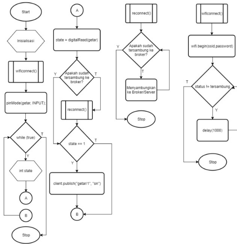
Gambar 4. Flowchart Pembacaan Data Sensor Getar
