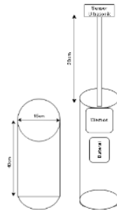
Gambar 10. Desain Patok/tiang Pembatas Sensor Ultrasonik
