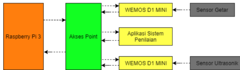
Gambar 1. Blok Diagram Sistem
