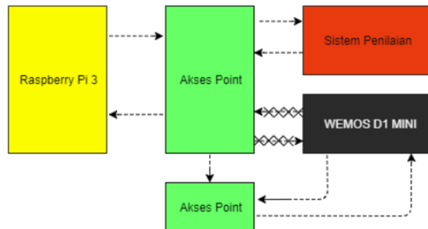
Gambar 8. Skema Jalur Koneksi Sistem dengan AP Tambahan
