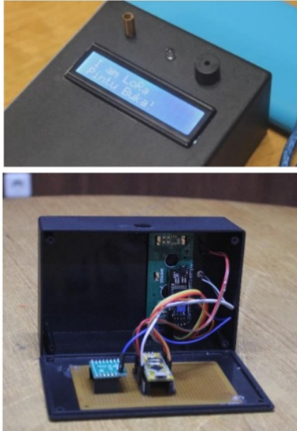
Gambar 2 Rangkaian Arduino dalam Box
