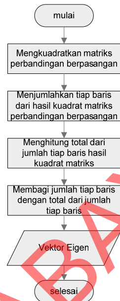
Gambar 5 Bagan Alir Proses Mencari Vektor Eigen Pada Metode AHP.
