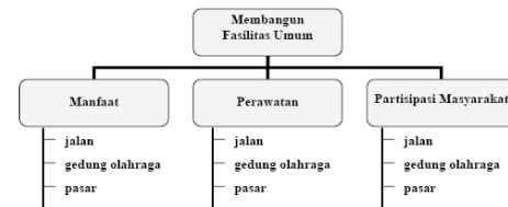
Gambar 2 Pohon Hierarki.
