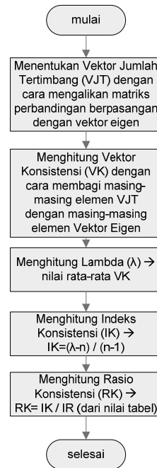
Gambar 6 Bagan Alir Proses Uji/Cek Konsistensi Pada Metode AHP.
