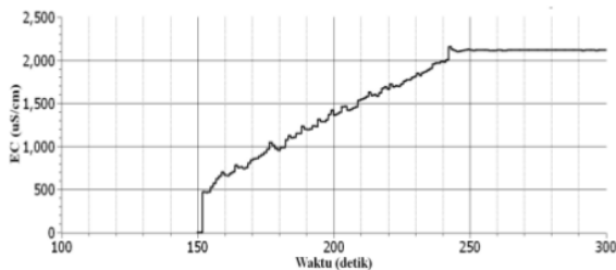
Gbr. 18 Grafik uji coba sensor EC dengan perlakuan ketiga dengan katup air membuka selama 150 detik.
