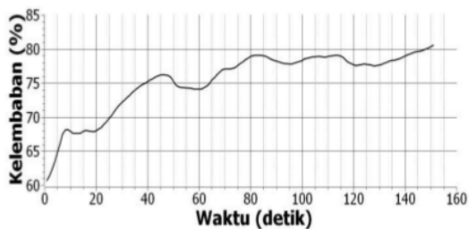
Gbr. 13 Grafik hasil uji coba kelembaban.
