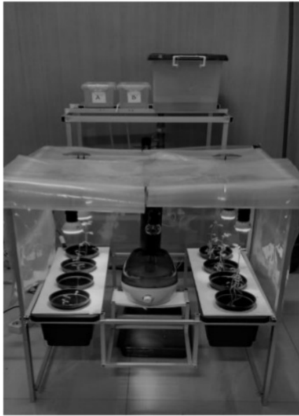
Gbr. 9 Sistem otomasi budidaya tanaman tomat ceri.
