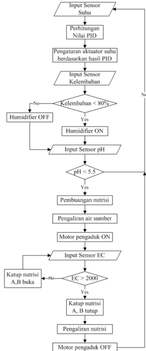
Gbr. 8 Diagram alir keseluruhan sistem.
