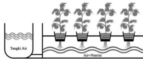
Gbr. 1 Sistem hidroponik wick .
