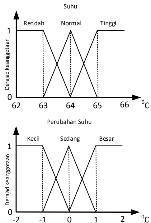
Gambar 7. Himpunan Fuzzy suhu dan perubahan suhu
