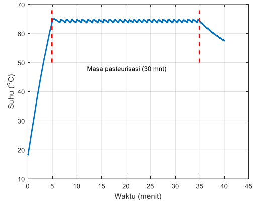
Gambar 6. Diagram respon waktu untuk proses pasteurisasi susu dengan pengendali PID
