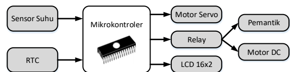
Gambar 2. Blok diagram sistem pasteurisasi susu
