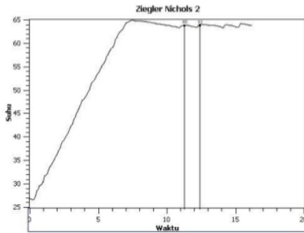
Gambar 5. Kurva respon dari sistem untuk nilai K_U = 53 .
