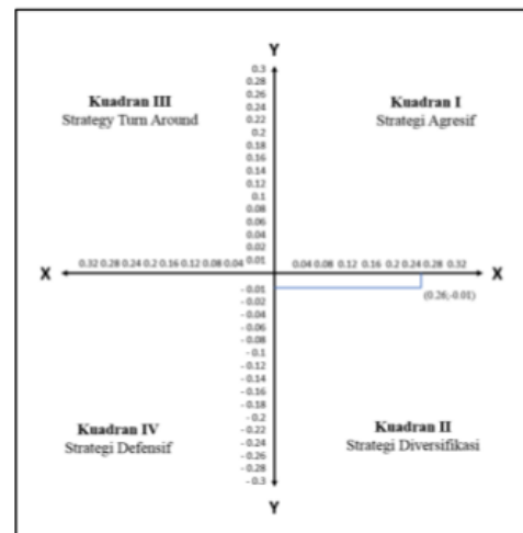
Gambar 3 Koordinat SWOT
