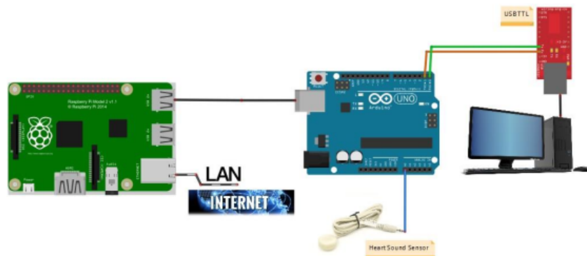
Gambar 2.3 Perancangan perangkat keras sistem monitoring IMedT
