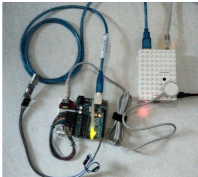
Gambar 3.1 Tampilan koneksi peralatan IMedT
