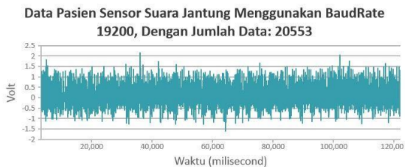
Gambar 5.1 Percobaan 1 pada Raspberry Pi 2 dengan baudrate 19200
