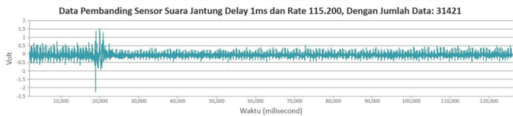
Gambar 5.10 PC pembanding dengan baudrate 115200 dan delay 1 milidetik
