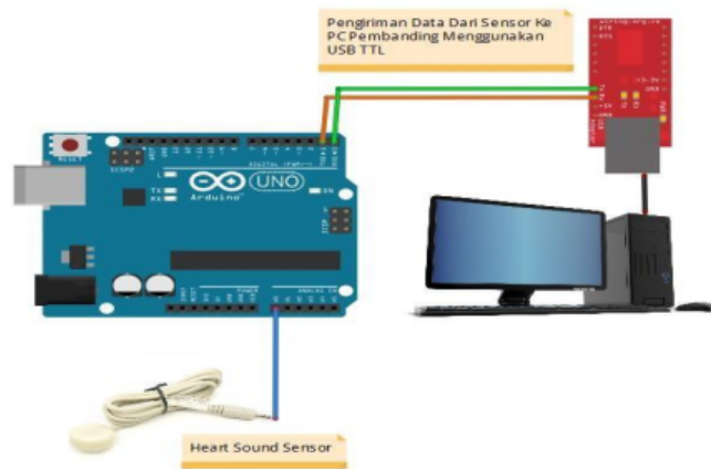
Gambar 2.8 Hubungan Arduino Uno dengan PC pembanding
