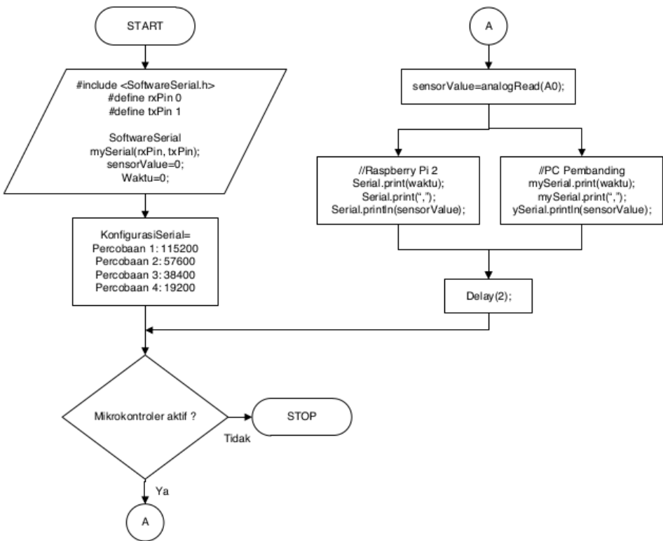
Gambar 2.10 Flowchart perbandingan bentuk sinyal auscultasi jantung
