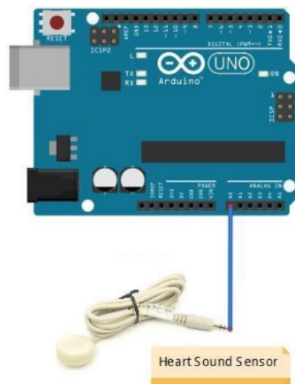
Gambar 2.5 Hubungan heart sound sensor dan Arduino.
