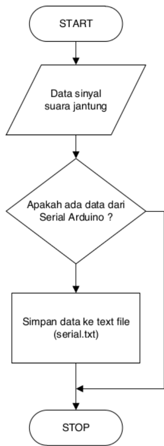
Gambar 2.12 Flowchart penerimaan data pada Raspberry Pi 2
