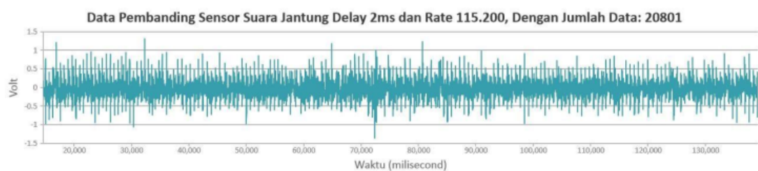
Gambar 5.12 PC pembanding dengan baudrate 115200 dan delay 2 milidetik
