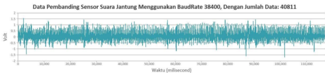
Gambar 5.4 Percobaan 2 pada PC pembanding dengan baudrate 38400
