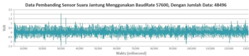
Gambar 5.6 Percobaan 3 pada PC pembanding dengan baudrate 57600
