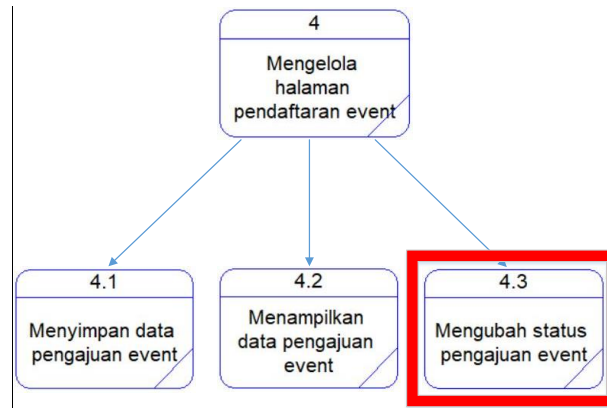
Gambar 4.7 Diagram Jenjang Level 1 Mengelola Halaman Pendaftaran Event
