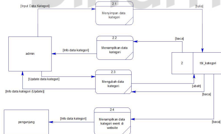
Gambar 4.22 DFD Level 2 Mengelola Halaman Kategori
