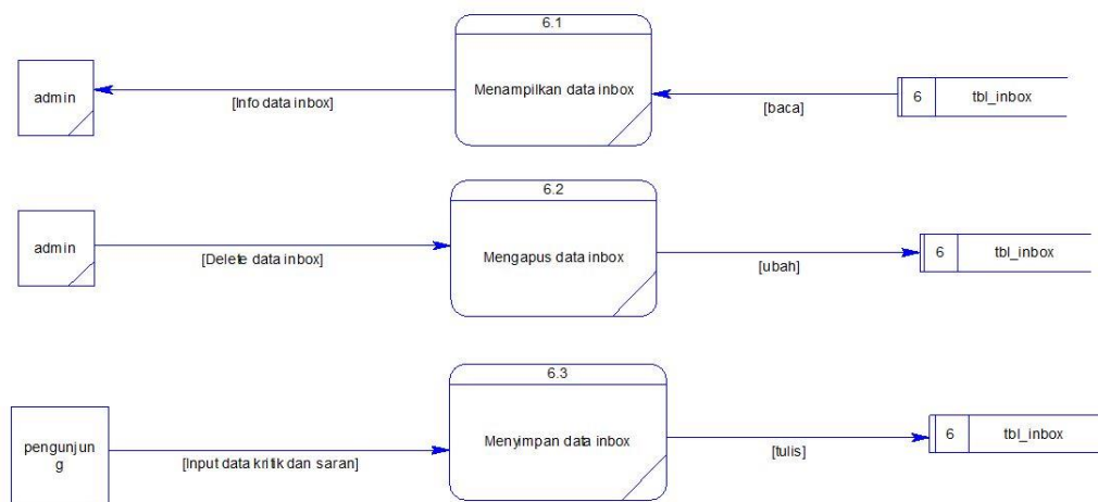
Gambar 4.26 DFD Level 2 Mengelola Halaman Inbox
