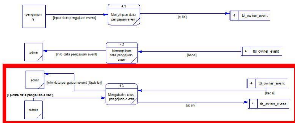
Gambar 4.24 DFD Level 2 Mengelola Halaman Pendaftaran event
