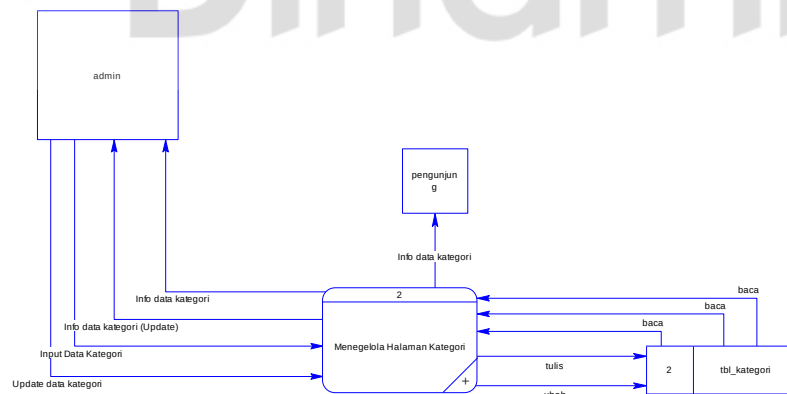
Gambar 4.14 DFD Level 1 Mengelola Halaman Kategori
