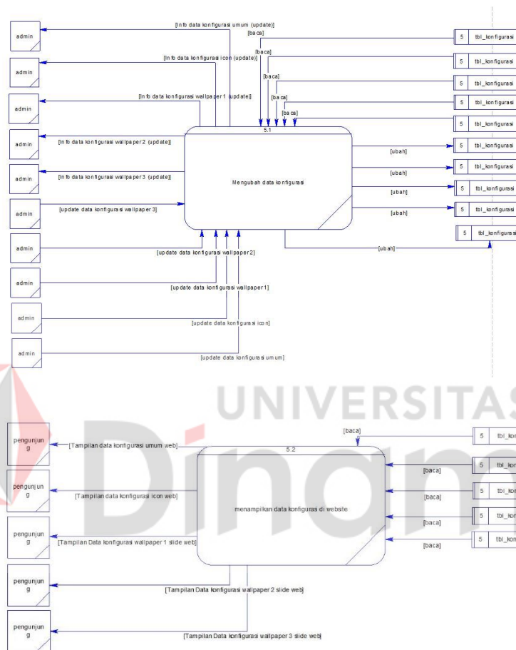
Gambar 4.25 DFD Level 2 Mengelola Halaman Konfigurasi
