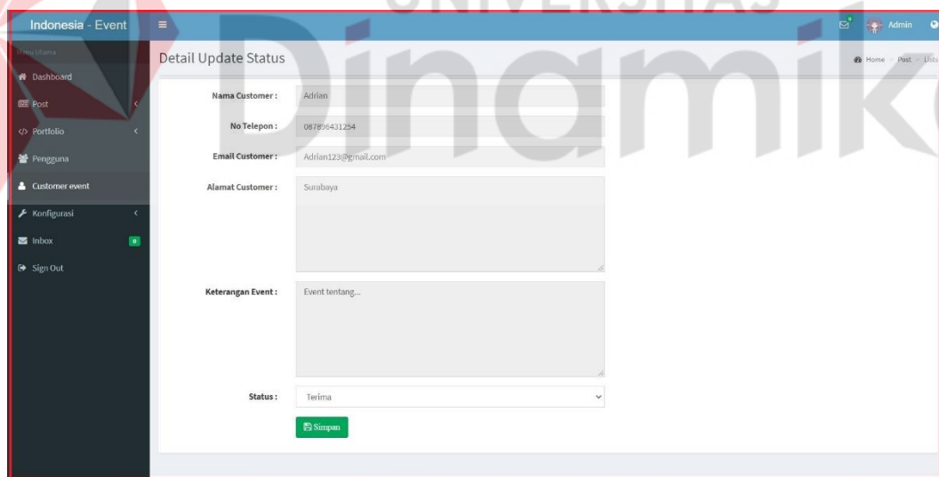
Gambar 4.46 Halaman Validasi
