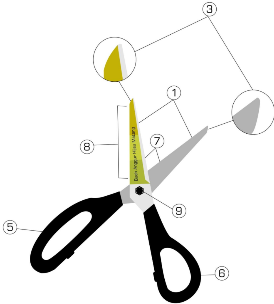
Gambar 2. Tampak Belakang 1 Gunting Panen Anggur Berwarna Sebagai Indikator Kematangan Buah
