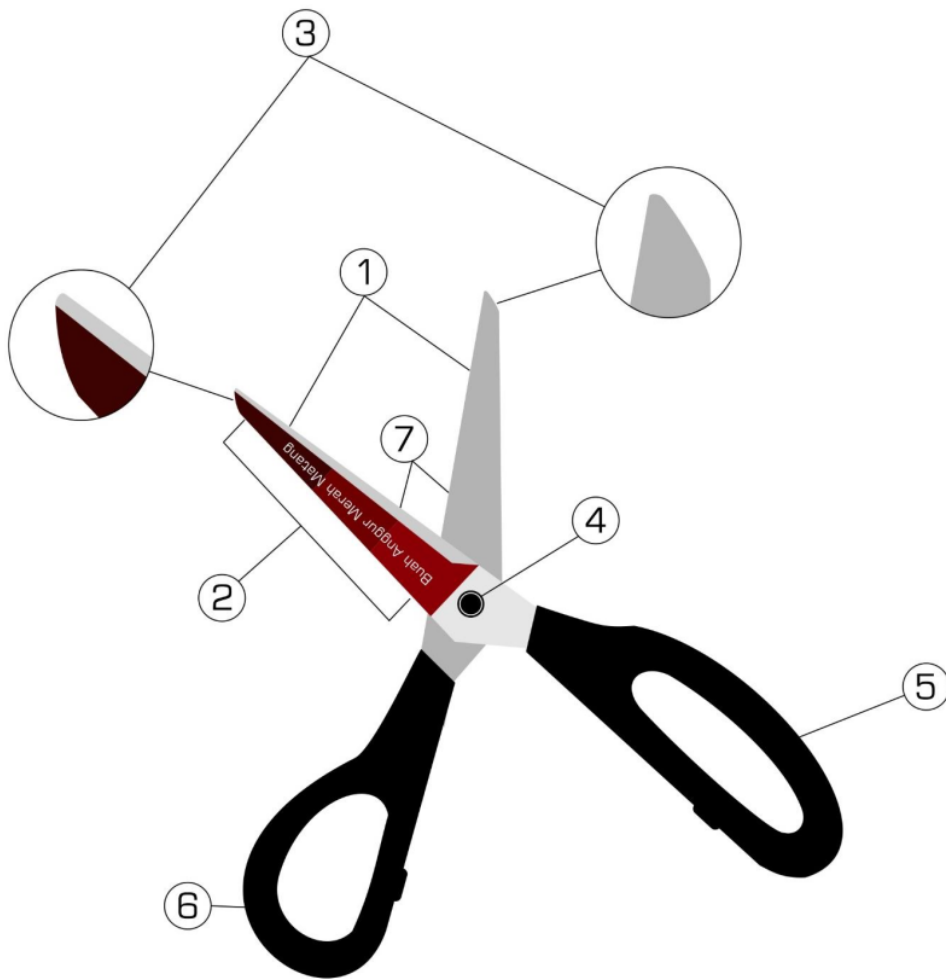
Gambar 1. Tampak Depan 1 Gunting Panen Anggur Berwarna Sebagai Indikator Kematangan Buah
