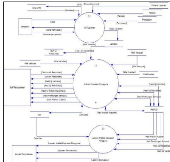
Gambar 2. DFD Sub Proses Analisis Kepuasan Pengguna
