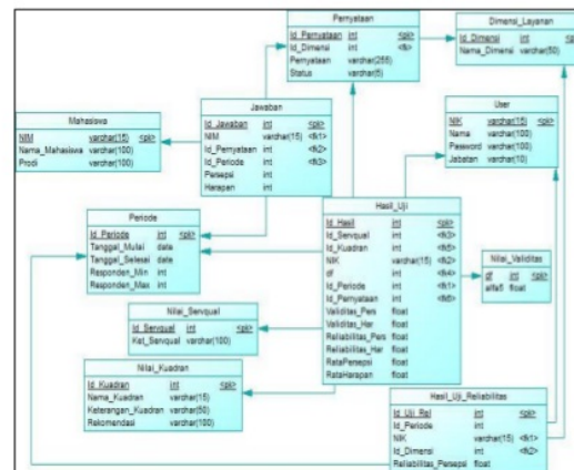
Gambar 3. Struktur Tabel
