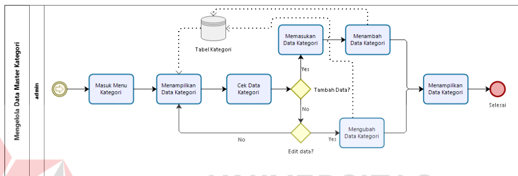
Gambar 1.5 Mengelola Data Master Kategori
