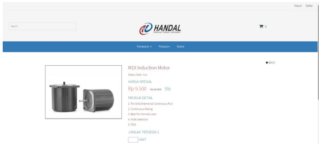
Gambar 3.3 Tampilan Produk
