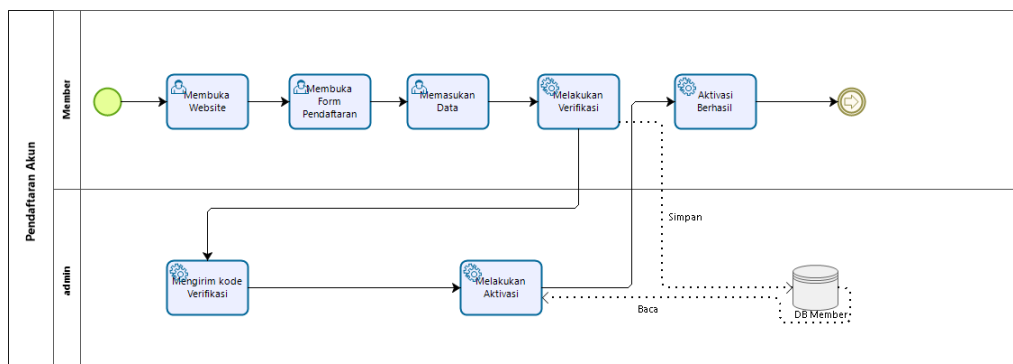
Gambar 1.7 Melakukan Pendaftaran
