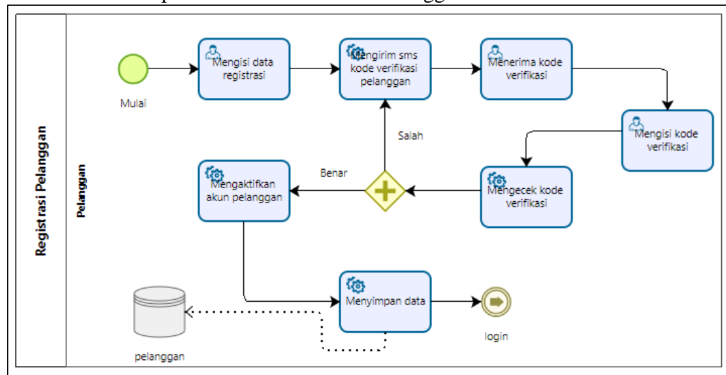
Gambar 1.2 Tampilan Daftar Akun User Pelanggan
