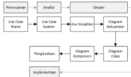
Gambar 6. Runut Balik Pemodelan Bisnis dengan UML dan SDLC
