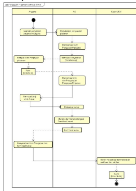
Gambar 9. Contoh Diagram Aktivitas Pengajuan Pinjaman
