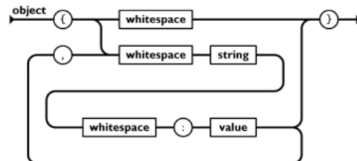
Gambar 1. JSON Object
