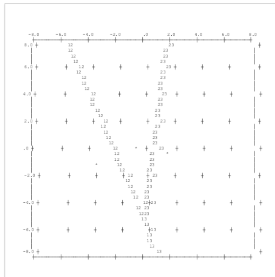
1 Kurang Baik; 2 Cukup Baik; 3 Baik *Indicates a group centroid Gambar 2 Territorial Map Capaian Penerapan PHBS
