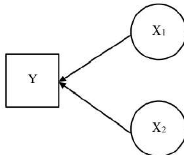
Gambar 1 Kerangka Konseptual
