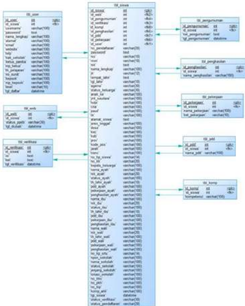
Gambar Lampiran 2 Physical Database Model dari aplikasi Pendaftaran
