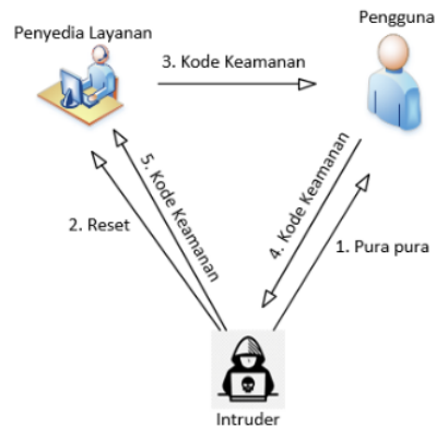
Gambar 4. Model 2FA dari Social Engineering berbasis SMS
