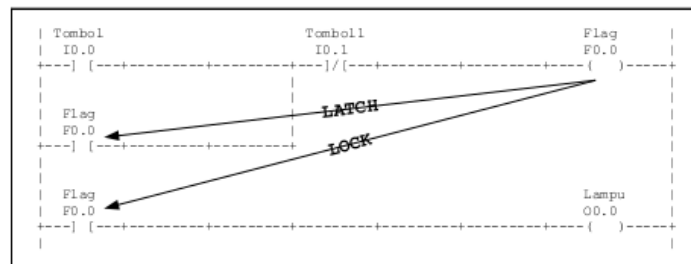
Gambar 3. Latch dan Lock sederhana
