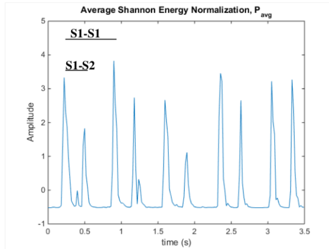
Gambar 7. Proses perhitungan waktu pada hasil Shannon Envelope
