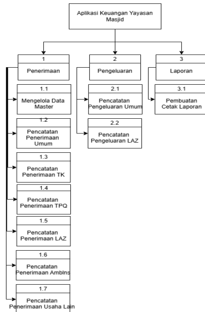
Gambar 2. 74 Diagram HIPO
