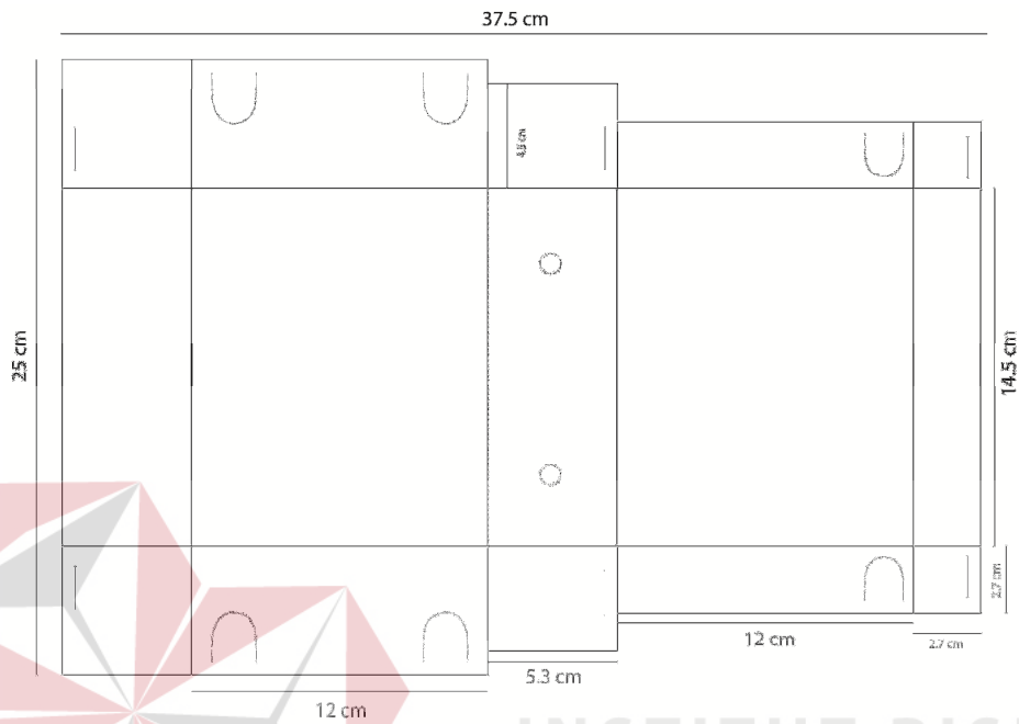
Gambar 3.5 Skema Beserta Ukuran Kemasan
