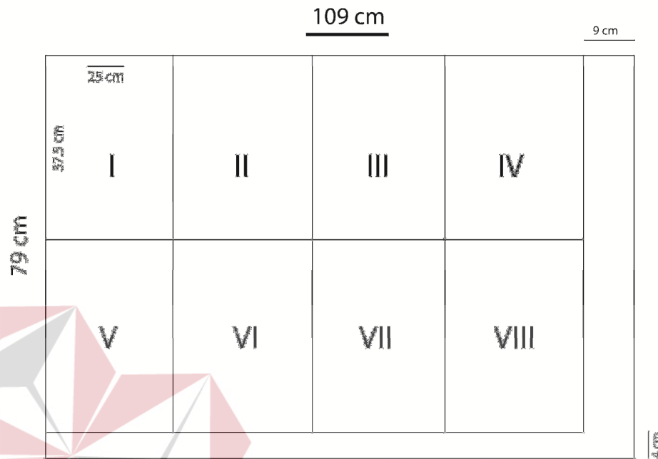
Gambar 3.6 Layout Potong Kertas
